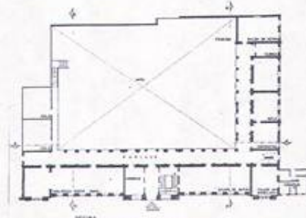
PLANTA BAJA DE LA ESCUELA SECUNDARIA N° 1, "CESAR A. RUIZ"
